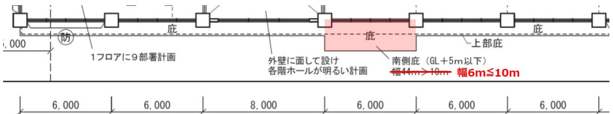
【基準階平面図（南側部分）】
