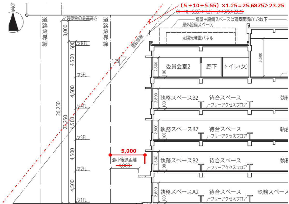
【断面図】
