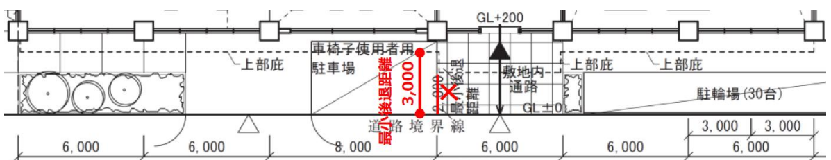
【1階平面図・配置図（南側部分）】
